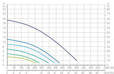
ATECF15 (1.5KW)
