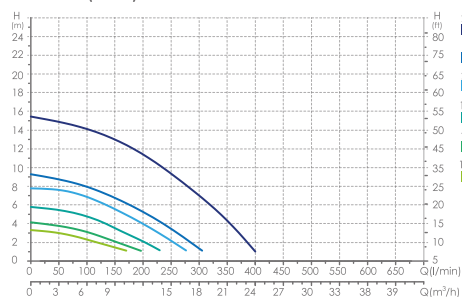
ATECF22 (2.2KW)
