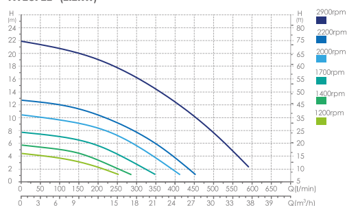
ATECF22 (2.2KW)
